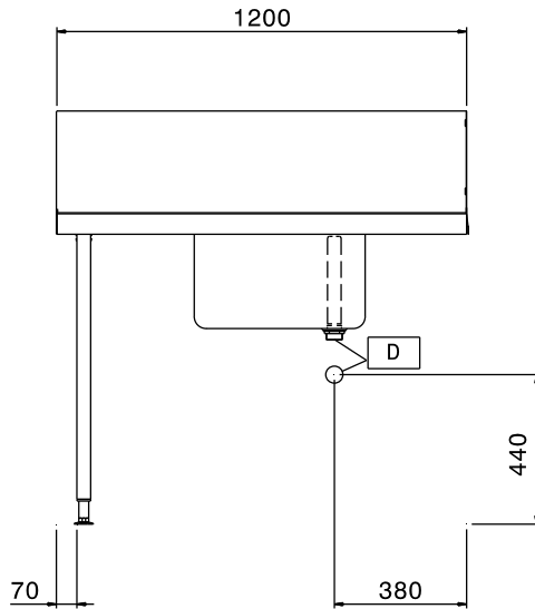
Front aanzicht
